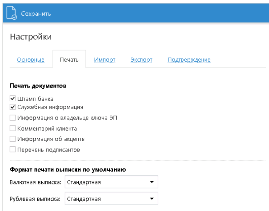
Рис. 7. Страница "Настройки". Закладка "Печать"
